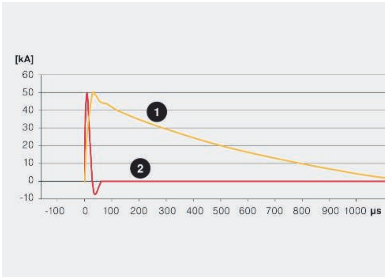
Vrste impulsa i njihove karakteristike: žuti = impulsna struja 1, direktan udar groma, 10/350-μs-simulirani impuls groma, crveni = impulsna struja 2, udaljeni udar groma ili preklonna operacija, 8/20-μs-simulirani impuls groma (prenapon)
