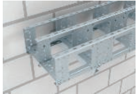
Mogelijke montagevariant van BKK-profiel met zijverbinding.
