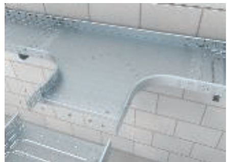
Montage T-Abzweigstück (Breite 400 - 600 mm)
